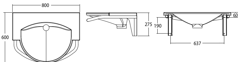
7201 Bano universaltvättställ med grått stödhandtag- med fasta monteringsfästen
