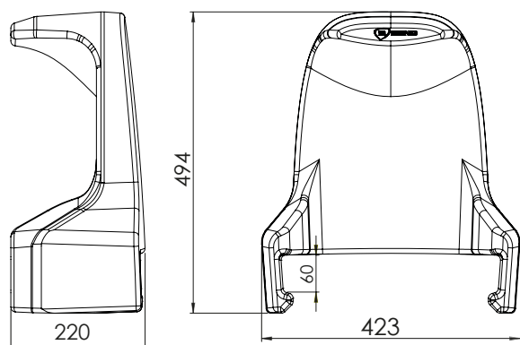
5972-03 Bano ryggstöd - grå Till 700 mm 5975 WC-skål
