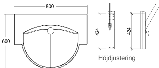
7202-02 Bano universaltvättställ med grått stödhandtag- med höjdjustering
