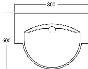
7200 Bano universaltvättställ utan stödhandtag- utan höjdjustering
